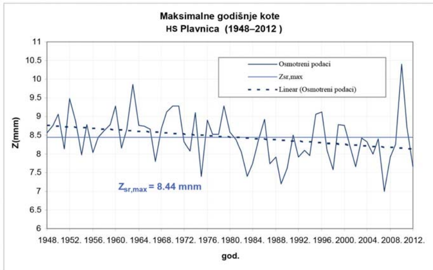
Grafikon 4.20 Analiza trenda maksimalnih godišnjih kote na HS Plavnica
