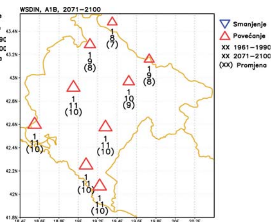
Grafikon 4.9b: Srednja godišnja vrijednost broja toplotnih talasa WSDIN tokom godine, za period 1961–1990. i prema scenariju A1B za period 2071–2100, sa promjenom ovog indeksa u odnosu na vrijednost iz perioda 1961–1990.
