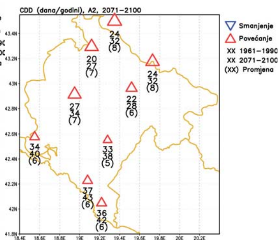
Grafikon 4.14b: Srednja godišnja vrijednost CDD indeksa za period 1961–1990. i prema scenariju A2 za period 2071–2100, sa promjenom ovog indeksa u odnosu na vrijednost perioda 1961–1990.
