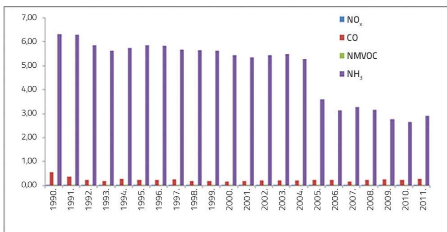
Grafikon 3.67: Ukupne indirektno GHG emisije iz sektora poljoprivrede, period 1990–2011. (Gg)
