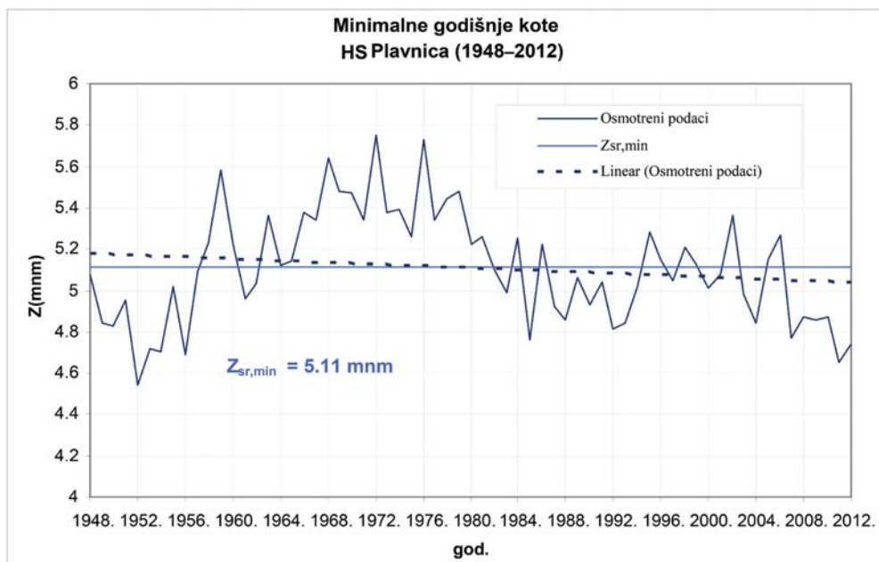
Grafikon 4.21 Analiza trenda minimalnih godišnjih kote na HS Plavnica
