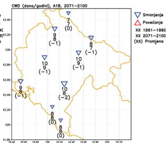
b) Grafikon 4.15b: Srednja godišnja vrijednost CWD indeksa za period 1961–1990. i prema scenariju A1B za period 2071–2100, sa promjenom ovog indeksa u odnosu na vrijednost iz perioda 1961–1990.
