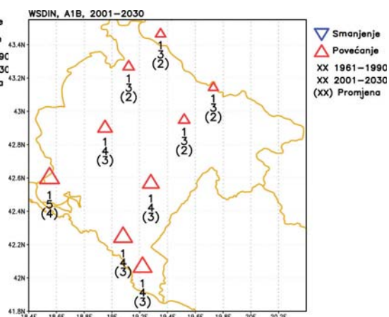
b) Grafikon 4.8b: Srednja godišnja vrijednost broja toplotnih talasa (WSDIN) tokom godine, za period 1961–1990. i prema scenariju A1B za period 2001–2030, sa promjenom ovog indeksa u odnosu na vrijednost iz perioda 1961–1990.
